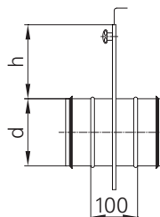
Rohrabsperrschieber Clapet à registre
