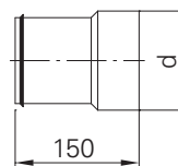
Schiebemuffe Manchon coulissant extérieur
